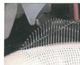
メリヤス編針の編成部
